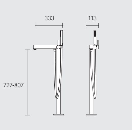
Смеситель для ванны, однорычажный
