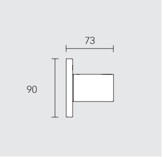
Вентиль-переключатель на 2 потребителя, для скрытого монтажа DN 15
