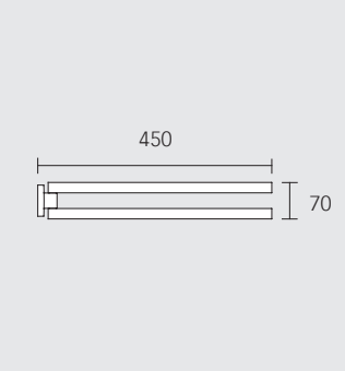
Полотенцедержатель двойной, поворотный
