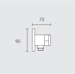
Соединение-вывод с держателем душевой лейки DN 15
