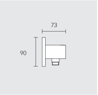
Соединение-вывод для шланга DN 15
