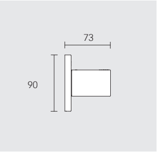
Запорный вентиль-переключатель на 3 потребителя, для скрытого монтажа DN 15
