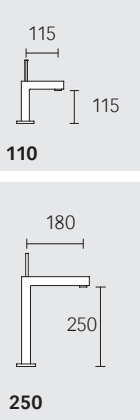
Смеситель для умывальника, однорычажный
