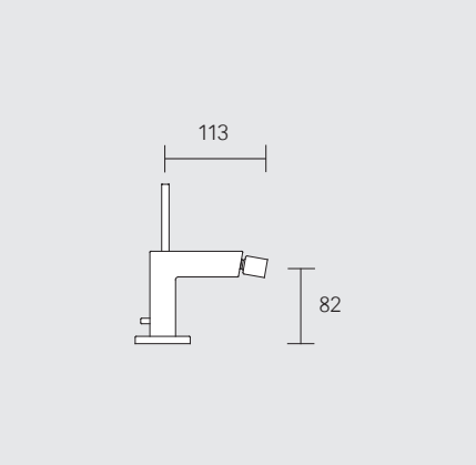
Смеситель для биде, однорычажный
