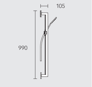
Душевой гарнитур серии
