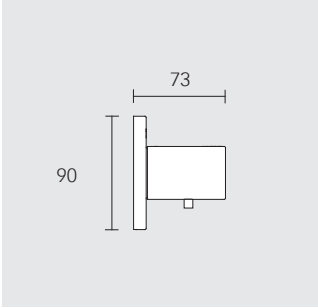
Термостат, для скрытого монтажа DN 15
