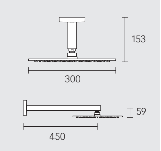
Верхний душ
