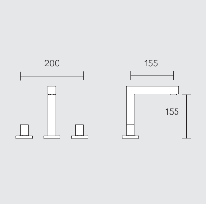
Смеситель для умывальника на три отверстия 150
