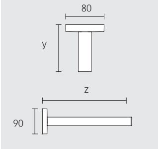
Душевой кронштейн DN 15
