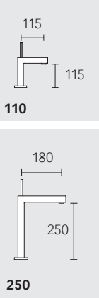
Смеситель для умывальника, однорычажный
