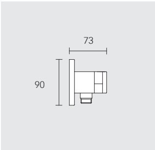
Przyłącze węża z uchwytem słuchawki prysznicowej DN 15 Gotowy zestaw do węży z nakrętką stożkową, samoistnie zabezpieczony przed przepływem wstecznym, według DIN EN 1717, pasuje do podtynkowego zestawu funkcyjnego 59547 000170 59092 010001
