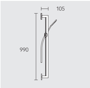
Zestaw prysznicowy Zawiera: drażek ścienny z uchwytem na słuchawkę prysznicową regulacja wysokości z uchwytem kąt nachylenia bezstopniowy regulowany, do wyboru w prawo lub w lewo płytkę porównawczą (5 mm) słuchawka prysznicowa ze strumieniem normalnym wąż prysznicowy, 1600 mm 59087 010001
