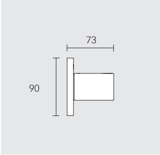
Dwudrożny zawór odcinająco-przestawny podtynkowy DN 15 Gotowy zestaw Zawiera: uchwyt, rozetę (okrągłą) i zawór odcinająco-przestawny pasuje do podtynkowego zestawu funkcyjnego 59556 000070 59057 010001
