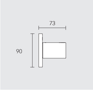
Dwudrożny zawór przestawny, podtynkowy DN 15 Gotowy zestaw Zawiera: uchwyt, rozetę (okrągłą) i zawór przestawny pasuje do podtynkowego zestawu funkcyjnego 59556 000070 59056 010001
