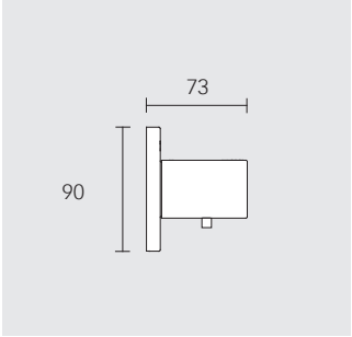
Bateria termostaticzna, podtynkowa DN 15 Gotowy zestaw Zawiera: uchwyt, rozetę (okrągłą) pasuje do podtynkowego zestawu funkcyjnego 59553 000070 59053 010001
