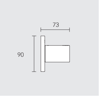
Zawór odcinający podtynkowy DN 15 Gotowy zestaw Zawiera: uchwyt, rozetę (okrągłą) i zawór odcinający pasuje do podtynkowego zestawu funkcyjnego 59541 000070 59041 010001
