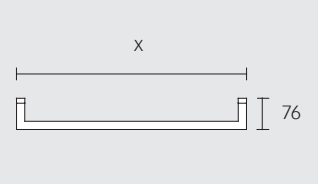
Reling na ręcznik Szerokość x: 560 / 760 mm 560 mm: 19101 010600 760 mm: 19101 010800
