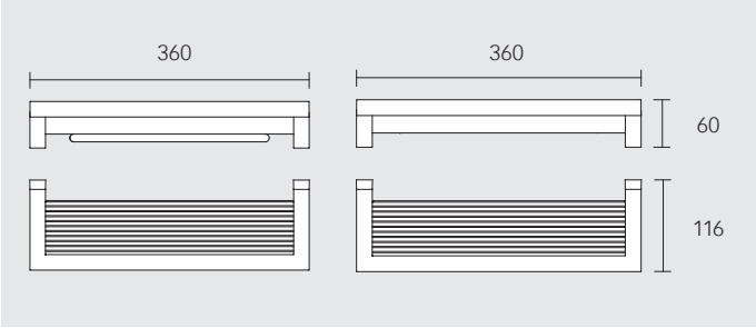
Półka prysznicowa • ze zintegrowaną ściągaczką wody lub bez • ściągaczka wody magnetyczna, jasnoszara (RAL 7035) ze ściągaczką wody: 19159 010000 chromowana / aluminium bez ściągaczki wody: 19158 010000 chromowana / aluminium
