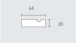
Haczyk na ręcznik pojedynczy 19114 010000
