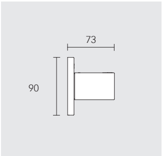
Trzydrożny zawór przestawny, podtynkowy DN 15 Gotowy zestaw Zawiera: uchwyt, rozetę (okrągłą) i zawór przestawny pasuje do podtynkowego zestawu funkcyjnego 59548 000070 59048 010001
