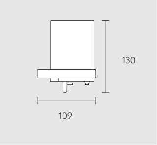
Dozownik do mydła kompletny ze szkła kryształowego Szkło kryształowe matowane, uchwyt i Pompa • ilość wypełnienia ok. 180 ml • ilość dozowania ok. 0,5 ml/skok 19152 019000
