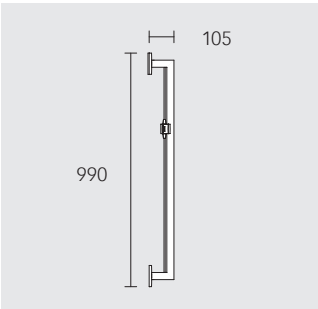
Drażek prysznicowy Zawiera: drażek ścienny z uchwytem na słuchawkę prysznicową regulacja wysokości z uchwytem kąt nachylenia bezstopniowy regulowany, do wyboru w prawo lub w lewo z płytką wyrównawczą (5 mm) 59085 010901
