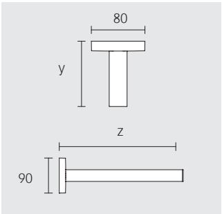
Ramię prysznica DN 15 Przyłącze sufitowe lub ściennie z okrągłą rozetą dekoracyjną Głębokość z: 319 / 469 mm Wysokość y: 100 / 300 mm Przyłącze sufitowe 100 mm: 59089 010101 300 mm: 59089 010301 Przyłącze ściennie 300 mm: 59088 010301 450 mm: 59088 010401
