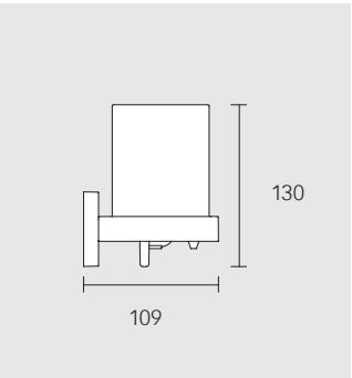
Dozownik do mydła kompletny ze szkła kryształowego Szkoło kryształowe matowane, uchwyt i pompa ilość wypełnienia ok. 180 ml ilość dozowania ok. 0,5 ml/skok 19052 019000
