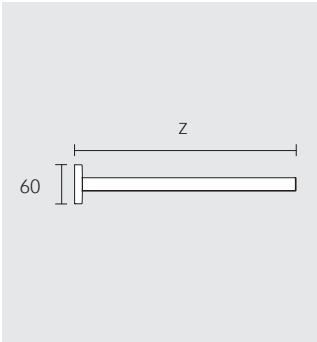
Wieszak na ręcznik 1-częściowy, stały Głębokość z: 340 / 450 mm 340 mm: 19022 010000 450 mm: 19020 010000
