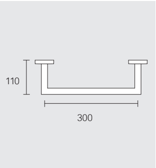
Obręcz na ręcznik stały 19021 010000
