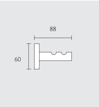
Haczyk na ręcznik podwójny 19015 010000
