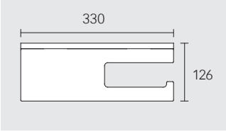
Uchwyt na papier toaletowy • z półką z przydymionego szkła • otwarty kształt • do szerokości rolki 100 / 120 mm 19173 018000
