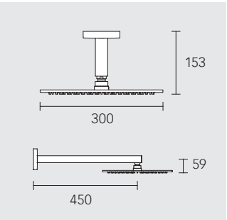
Deszczownica Przyłącze sufitowe lub ściennie z okrągłą rozetą dekoracyjną Ilość przepływu ograniczona do 15 l / min. Deszczownica ø 300 mm, G 1/2 (59986 010301) Przyłącze sufitowe 59084 010101 Przyłącze ściennie 59083 010401
