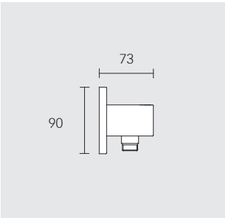
Przyłącze węża DN 15 Gotowy zestaw do węży z nakrętką stożkową, samoistnie zabezpieczony przed przepływem wstecznym, według DIN EN 1717, pasuje do podtynkowego zestawu funkcyjnego 59547 000170 59047 010001
