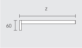
Wieszak na ręcznik 1-częściowy, stały Głębokość z: 346 / 456 mm 346 mm: 19122 010000 456 mm: 19120 010000
