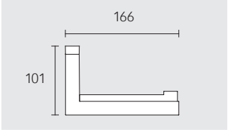
Uchwyt na papier toaletowy • otwarty kształt, z hamulcem rolki • do szerokości rolki 100 / 120 mm 19162 010000
