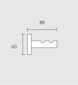
Handdoekhaak dubbel 19015 010000
