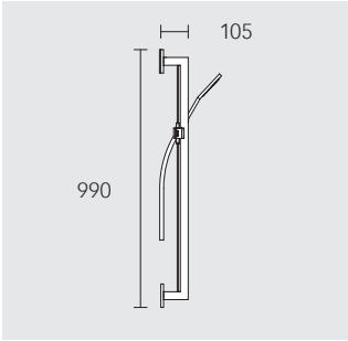
Douchestangset Bestaande uit: Muursteen met hand-douchegeleider In hoogte verstelbaar Hellingshoek traploos verstelbaar, naar keuze rechts of links Met tegelopvulstuk (5 mm) Handdouche met 1 straal Doucheslang 1600 mm 59087 010001
