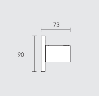
Stopkraan UP DN 15 Kant-en-klare set Bestaande uit: Greep, rozet (rond) en stopkraan passend voor UP functie-eenheid 59541 000070 59041 010001
