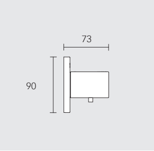
Thermostaatarmatuur UP DN 15 Kant-en-klare set Bestaande uit: Greep, rozet (rond) passend voor UP functie-eenheid 59553 000070 59053 010001
