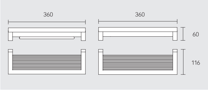
Doucheplanchet
