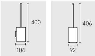
Toiletborstelgarnituur
