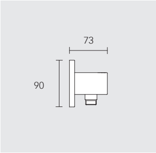
Slangaansluiting DN 15 Kant-en-klare set voor slangen met conische moer, Intrinsiek veilig tegen terugstromen, conform DIN EN 1717, passend voor UP functie-eenheid 59547 000170 59047 010001
