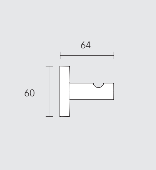
Handdoekhaak enkel 19014 010000
