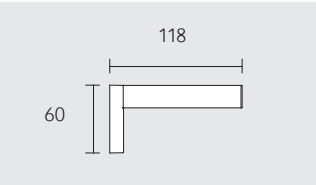
Toiletpapier- reserverolhouder
