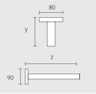
Douchearm DN 15 Plafond- of wandaansluiting met ronde rozet Diepte z: 319 / 469 mm Hoogte y: 100 / 300 mm Plafondaansluiting 100 mm: 59089 010101 300 mm: 59089 010301 Wandaansluiting 300 mm: 59088 010301 450 mm: 59088 010401
