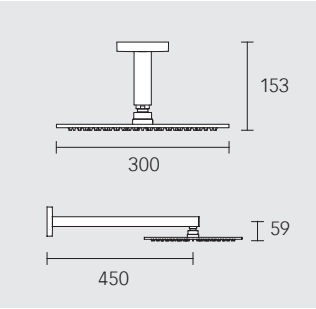
Hoofdsproeier Plafond- of wandaansluiting met ronde rozet doorstroomhoeveelheid begrensd op 15 l/min. Hoofdsproeier ø 300 mm, G 1/2 (59986 010301) Plafondaansluiting 59084 010101 Wandaansluiting 59083 010401
