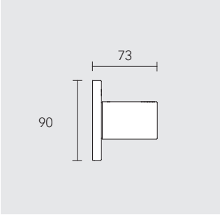
2-weg instelventiel UP DN 15 Kant-en-klare set Bestaande uit: Greep, rozet (rond) en instelventiel passend voor UP functie-eenheid 59556 000070 59056 010001
