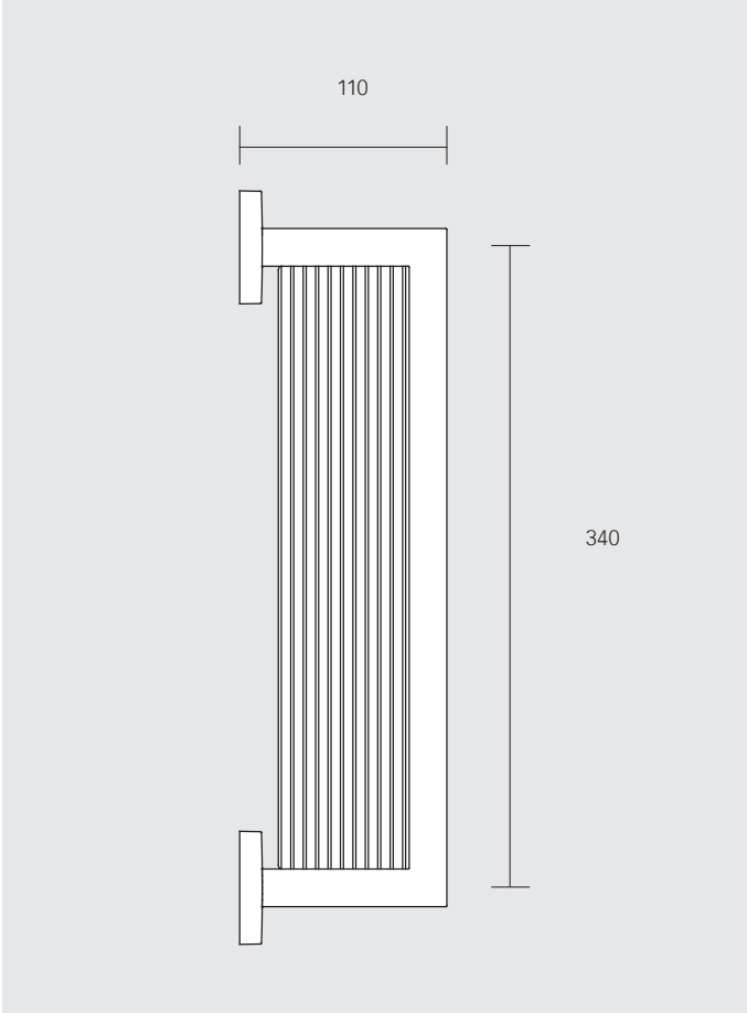
Doucheplanchet met of zonder geïntegreerde wisser wisser magnetisch, lichtgrijs (RAL 7035) met wisser: 19059 010000 verchroomd/aluminium zonder wisser: 19058 010000 verchroomd/aluminium
