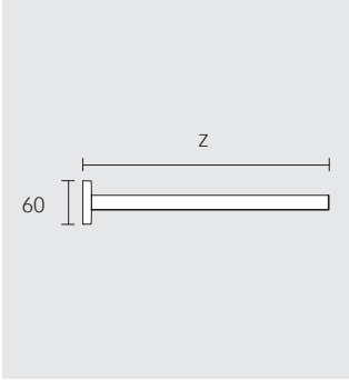
Handdoekhouder 1-delig, vaststaand Diepte z: 340 / 450 mm 340 mm: 19022 010000 450 mm: 19020 010000
