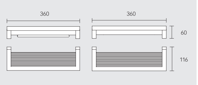
Mensola per doccia
