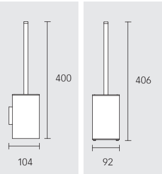
Portascopino ▪ contenitore in plastica antracite ▪ spazzola con asta e scovolo di ricambio nero 19064 010101 Modello a muro 19069 010100 Modello da terra
