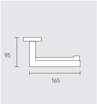
Portarotolo ▪ aperto, con fermo rotolo ▪ per larghezza del rotolo 100 / 120 mm 19062 010000
