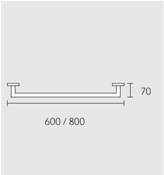
Portasalviette Larghezza x: 600 / 800 mm 600 mm: 19001 010600 800 mm: 19001 010800
