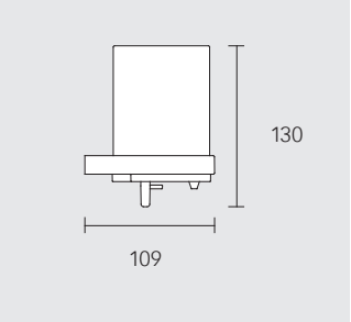
Spandisapone completo con vetro in cristallo satinato
