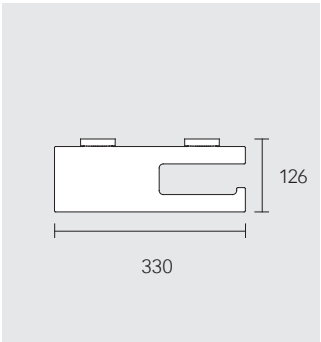
Portarotolo ▪ con ripiano in vetro fumé ▪ aperto ▪ per larghezza del rotolo 100 / 120 mm 19073 018000
