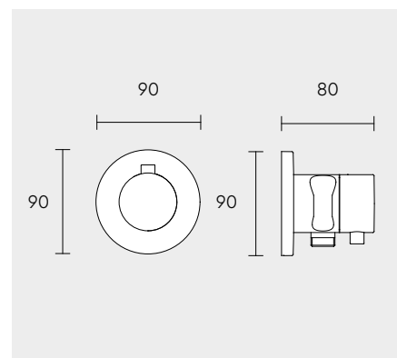
Thermostatarmatur Set Unterputz für 2 Verbraucher mit Schlauch- anschluss und Brausehalter
