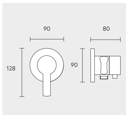
Einhebelmischer Set Unterputz für 2 Verbraucher mit Schlauch- anschluss und Brausehalter
