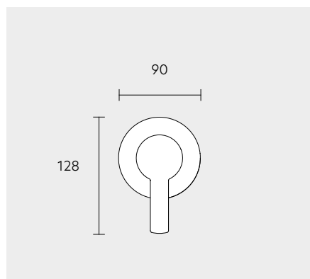
Einhebelmischer Unterputz PLAN blue
