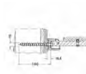
Befestigungs-Set 6 Seite 404
