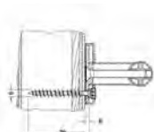
Befestigungs-Set 4 Seite 404
