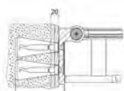
Befestigungs-Set 10 Seite 402
